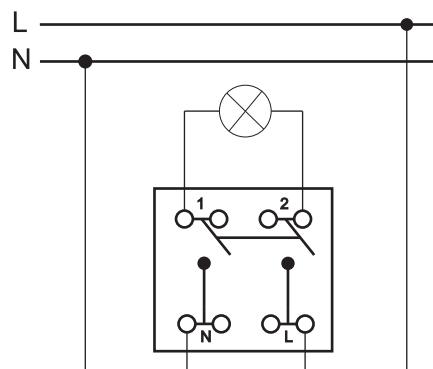
Schemat podłączenia łącznika dwubiegunowego.
